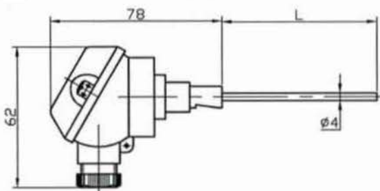
Рисунок 1. Внешний вид термопреобразователя сопротивления ТСП-Н комплекта.
